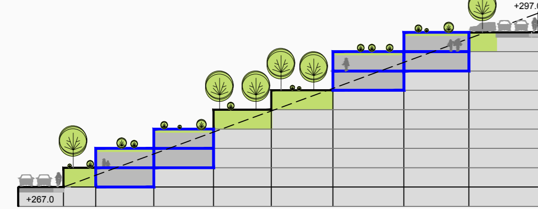
KARAKTERISTIČAN PRESJEK (moguće oblikovanje građevina)
