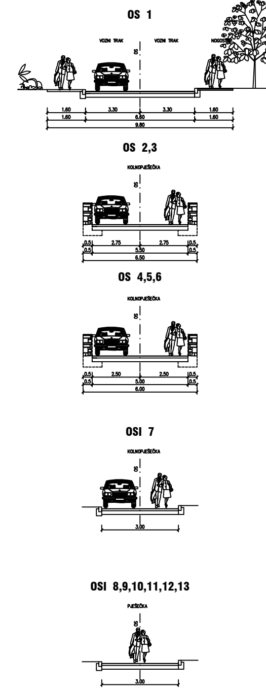
KARAKTERISTIČNI POPREČNI PROFILI UPU RUSKAMEN
